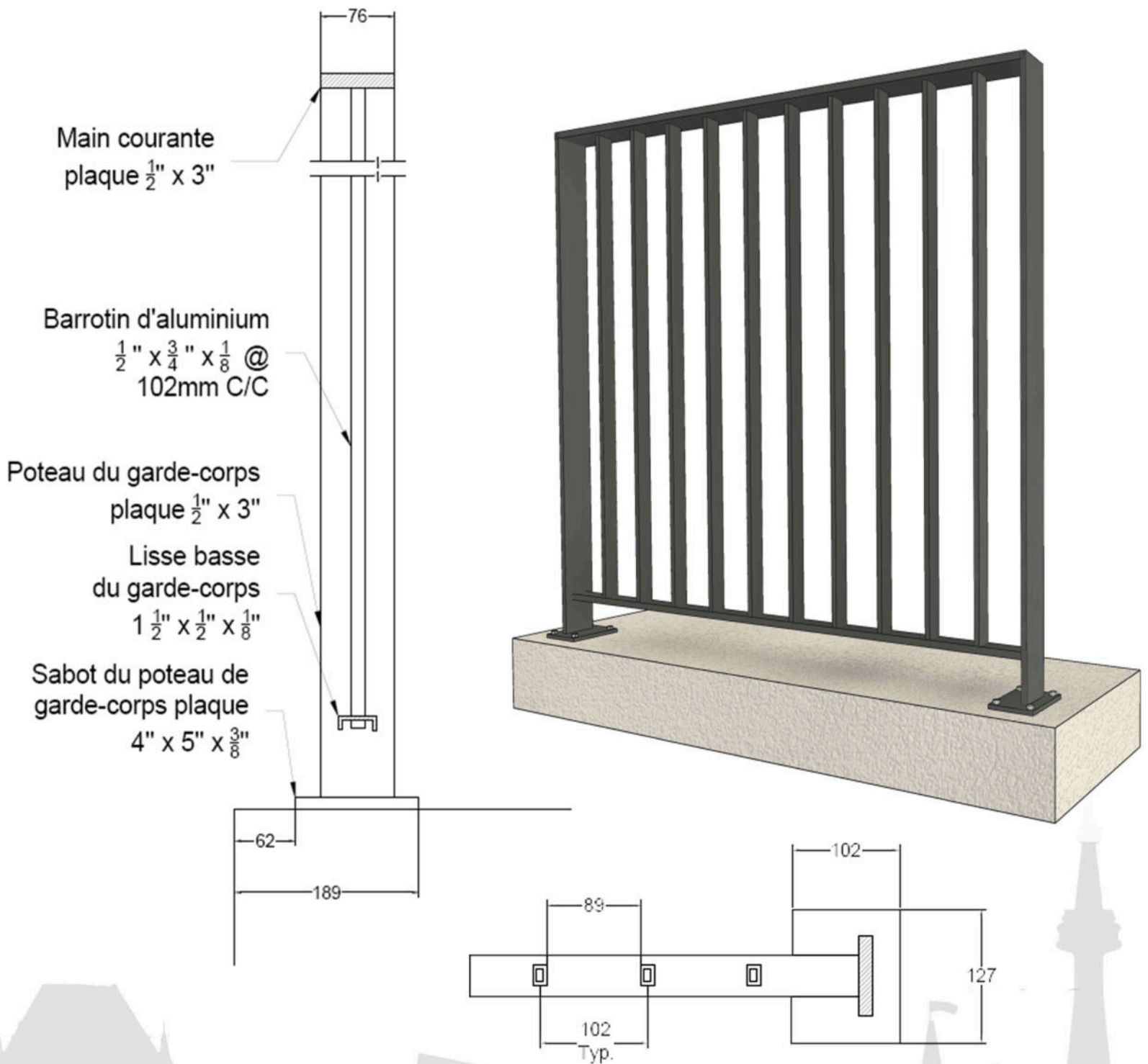
DÉTAIL DE BASE
