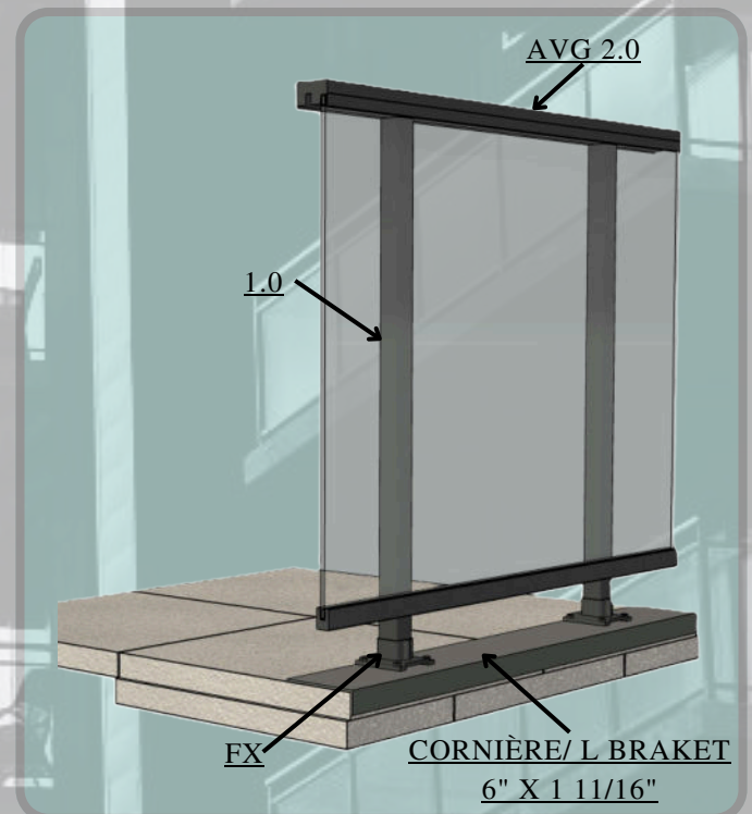
VITRÉ FAÇADE SUR PLOT GLASS FACADE ON PEDESTAL
